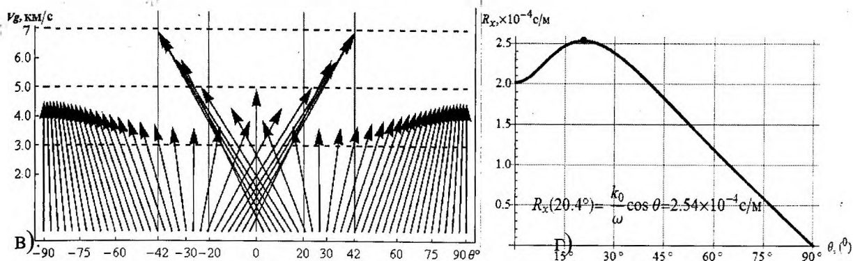
а) нормали к поверхности обратных скоростей; б) значения групповой скорости; в) векторная диаграмма сноса групповой скорости от угла направления; г) в точке R_{xmax} групповая скорость направлена вдоль оси X
