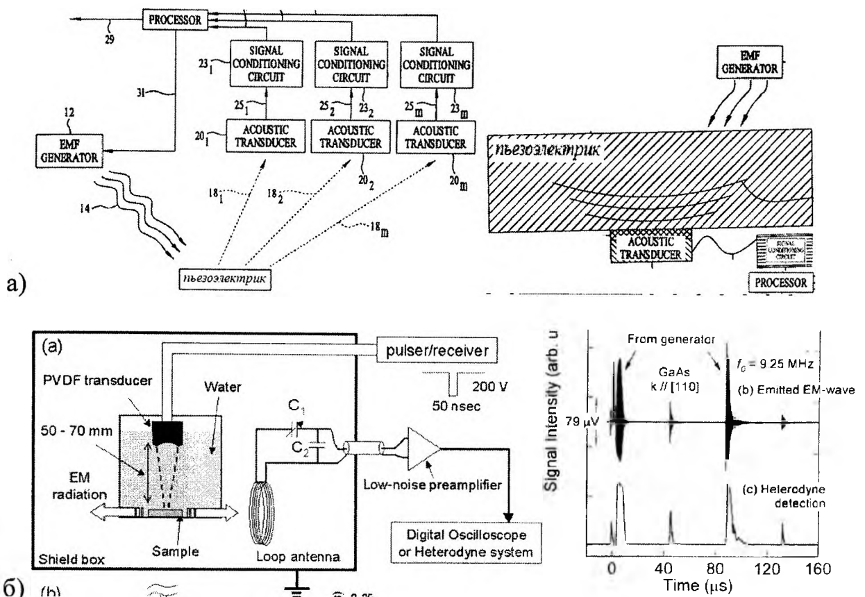
а) схема для анализа свойств пьезоэлектрика с помощью упругой волны порожденный ЭМ волной [26]; б) детектирование электромагнитной волны от воздействия ультразвука на пьезоэлектрик [19, 20]
