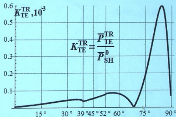
Рисунок 3.15 – Коэффициент трансформации энергии SH волн в электромагнитную
