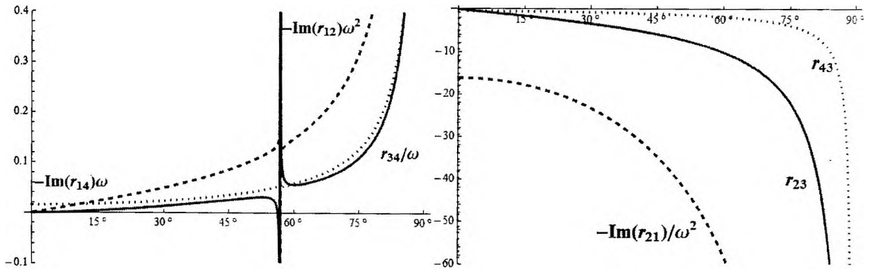
Рисунок 3.17 – График зависимостей элементов матрицы \mathbf{R} от значения угла \theta для анизотропных параметров (KNbO3)
