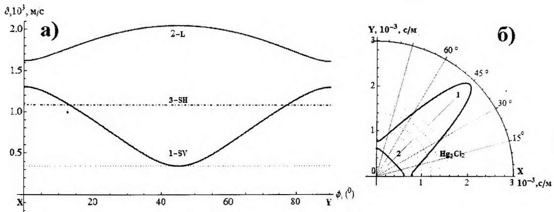
а) скорости упругих волн; б) поверхности волновых векторов; 1 – для SV волны, 2 – для продольной волны
