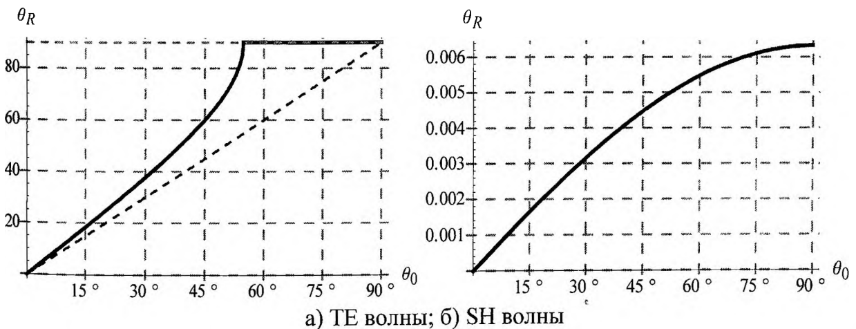
Рисунок 3.3 – по абсциссе углы падения ТЕ электромагнитной волны, по ординате соответствующие углы преломления (в градусах)
