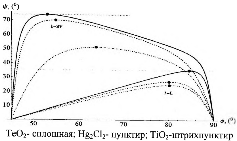
Рисунок 2.8 – Значения угла сноса поперечной (1-SV) и продольной (2-L) волны от угла падения
