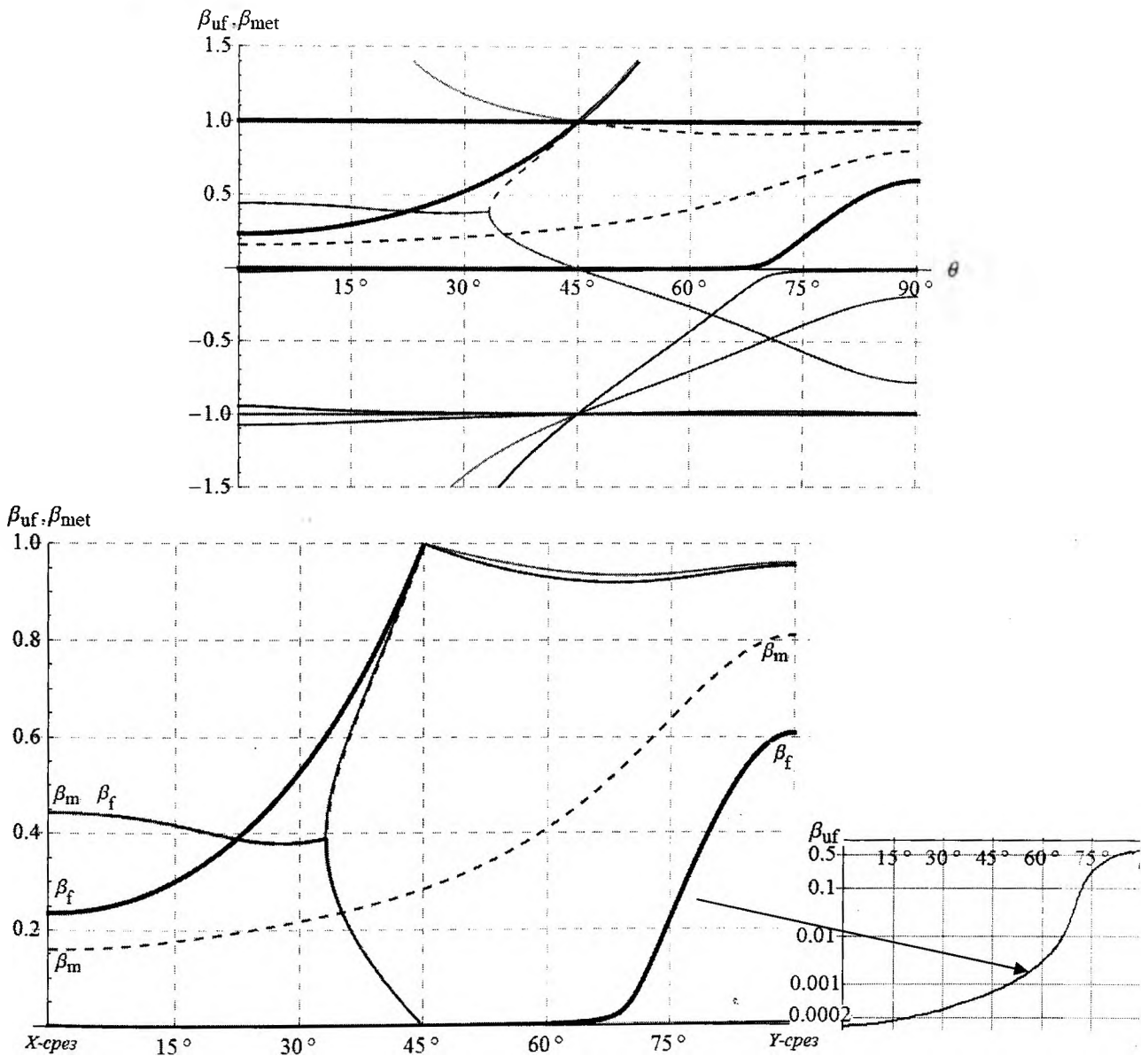
Рисунок 4.2 – Изменение показателя спадания волн Г-Б для ниобата калия. Срез меняется перпендикулярно оси Z (XOY)
