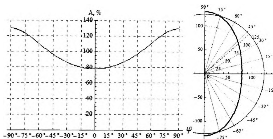
Рисунок 2.15 – Распределение плотности потока энергии в XOY плоскости для \text{KTiOAsO}_4
