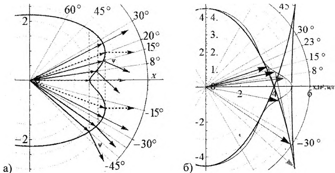
Рисунок 2.11 – Направления групповой скорости SH волн в \text{KNbO}_3 , лист 1
