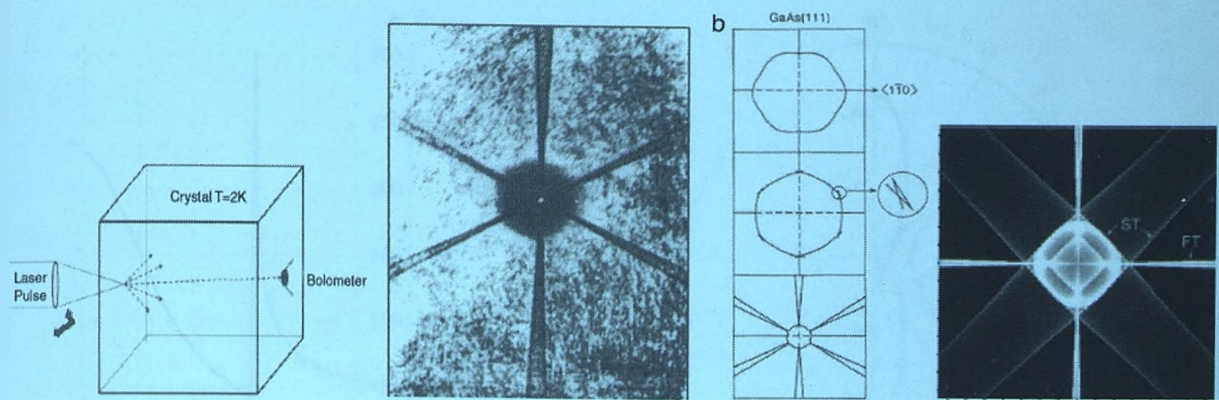
Рисунок 2.13 – Экспериментальное наблюдение фононной фокусировки упругих волн в кубическом кристалле GaAs (111) и в Si (001) [112]
