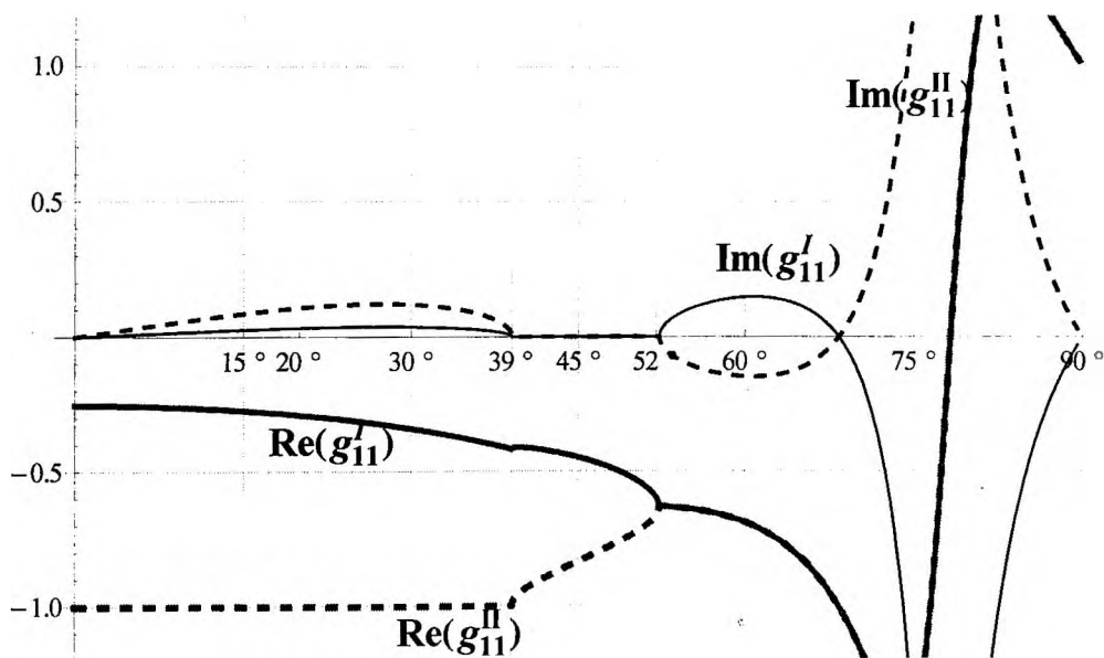
Рисунок 3.19 – График зависимостей элементов матрицы \mathbf{G} от угла \theta (к задаче двойного лучепреломления без изменения ветви), лист 1
