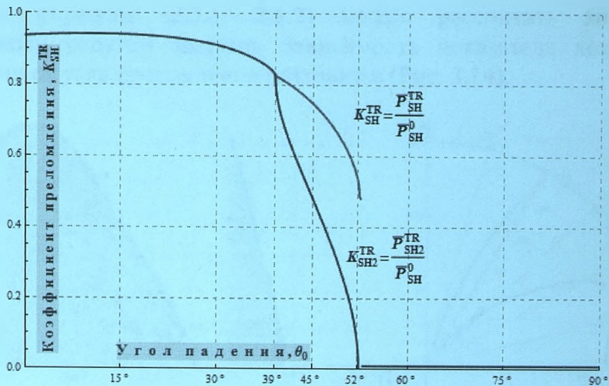
Рисунок 3.12 – Коэффициент преломления фазового волнового фронта упругой SH волны от границы изотропный диэлектрик-пьезоэлектрик \text{KNbO}_3
