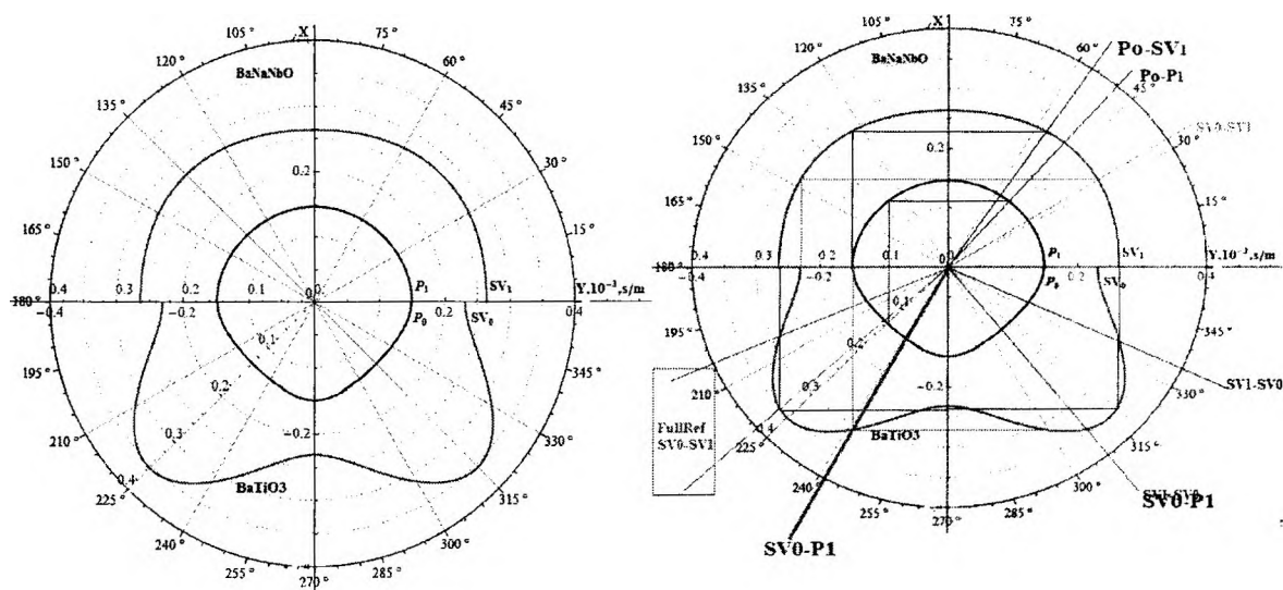
Рисунок 3.4 – Поверхности волновых векторов P, SV волн для \text{BaTiO}_3 и \text{Ba}_2\text{NaNb}_5\text{O}_{15} . Графическое определение углов отражения и преломления в зависимости от типа падающей волны
