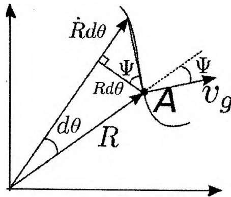
Рисунок 2.7- Графическая иллюстрация для определения угла сноса
