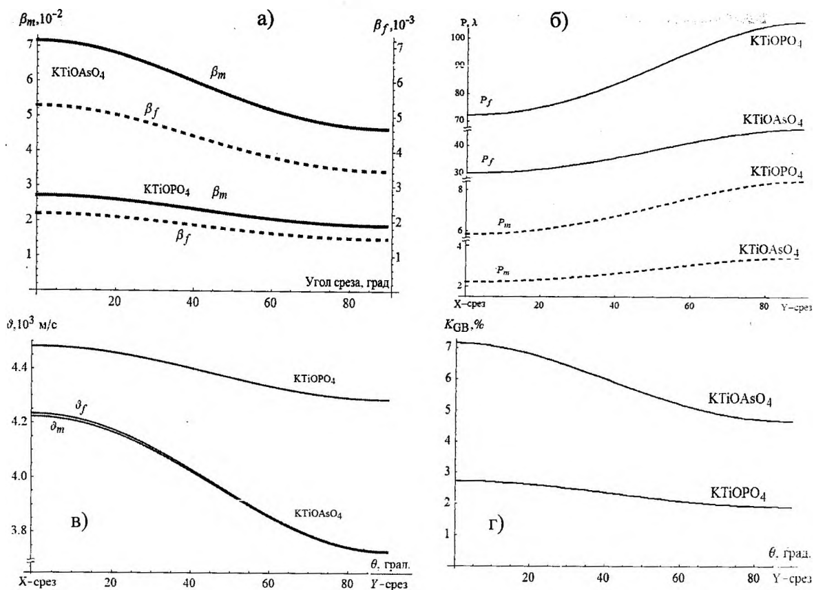
Рисунок 4.3 – Характеристики волн Г-Б для \text{KTiOAsO}_4 и \text{KTiOPO}_4
