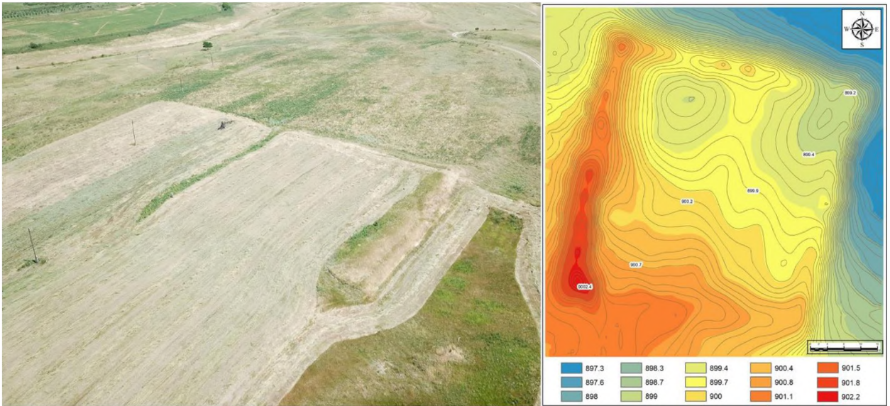
9-сурет. Бактай төрткүлі. Өуеден түсірілген фотосуреті мен топографиялық жоспары
