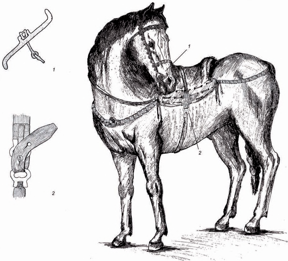
Рис. 14. Акжайлау, курган № 1. Графическая реконструкция снаряжения верховой лошади: 1 – соединение бронзовых удил и железных псалиев; 2 – соединение подпружных ремней. Реконструкция авторов. Художник – Адилхан Рахметов
