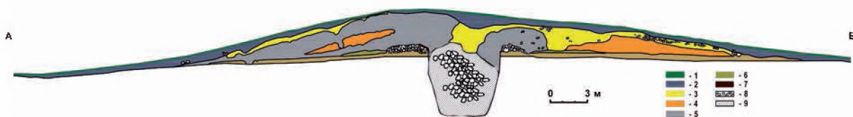
Рис. 4. Акжайлау, курган № 1. Разрез: 1 – дерн; 2 – гумус; 3 – смешанный слой; 4 – глина светло-коричневого цвета; 5 – основная насыпь; 6 – выкид из могильной ямы; 7 – дерево; 8 – камни; 9 – заполнение могильной ямы. Исполнитель: Максим Половцев
