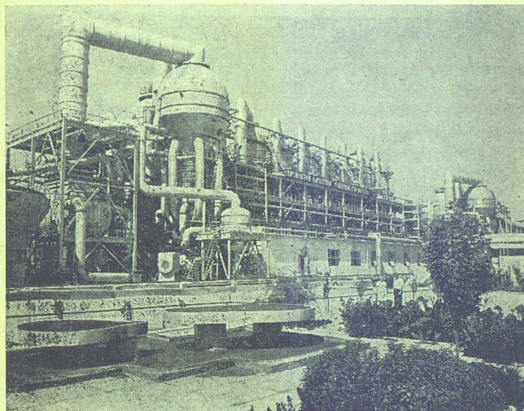
Су тұщытатын атом қондырғысының сыртқы көрінісі
