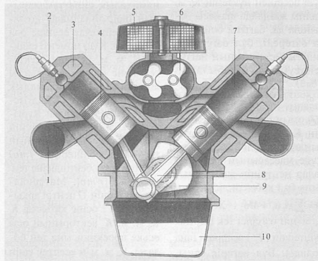
Дизельді қозғалтқыш: 1 — газ шығару келтеқұбыры (патрубок); 2 — бүріккіш (форсунка); 3 — салқындатқыш су; 4 — піспек (поршень); 5 — ауа сүзгі; 6 — ауа қысып тығыздағыш; 7 — цилиндр; 8 — бұлғақ (шатун); 9 — иінді білік; 10 — май шомылғышы.
